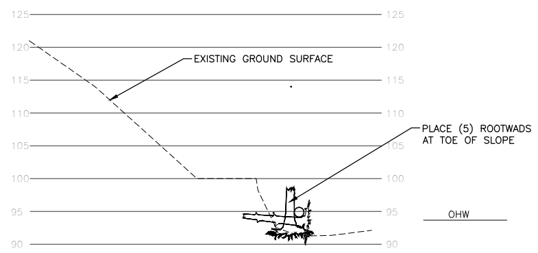
SECTION SCALE: 1" = 20'
